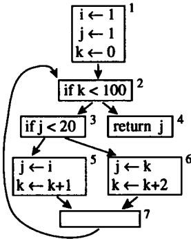
(b) CFG
